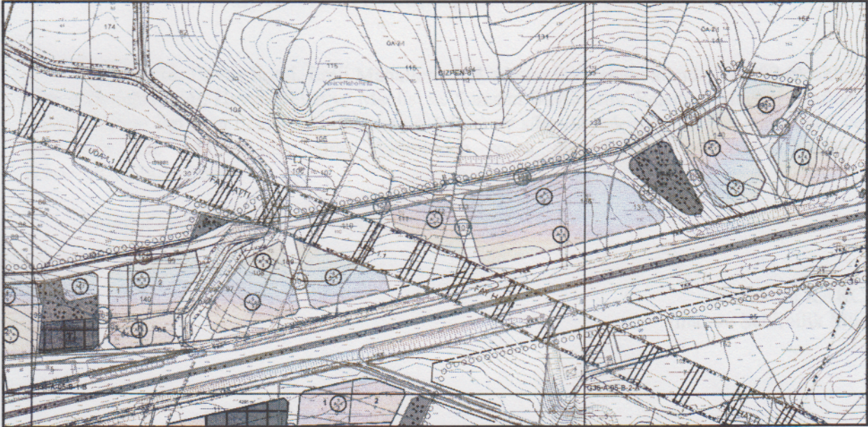
ERELİ MAHALLESİ UYGULAMA ALANI, MEVCUT UYGULAMA İMAR PLANI
