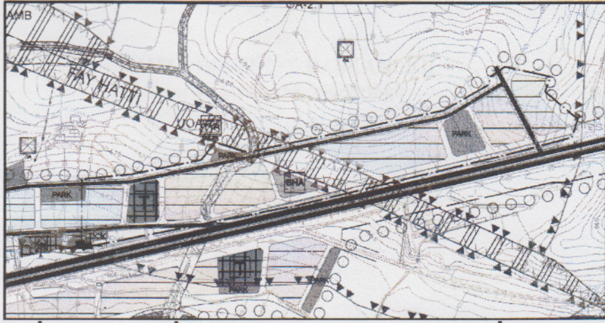
ERELİ MAHALLESİ UYGULAMA ALANI, NAZİM İMAR PLANI
